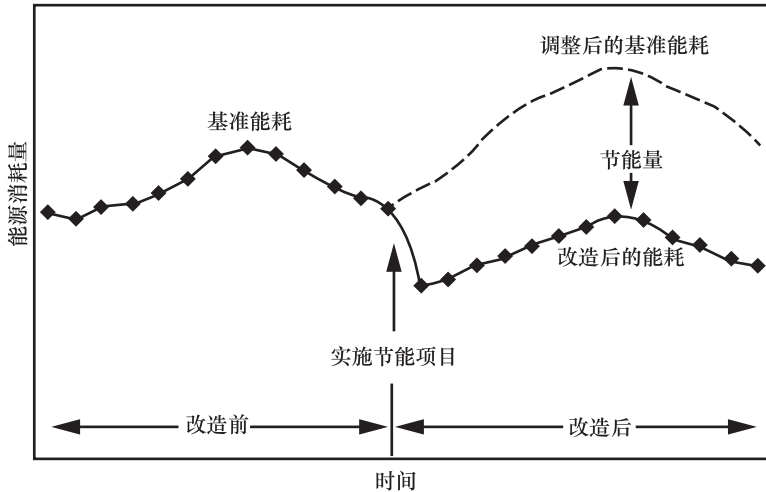
图 12-1 节能量的确定方法
